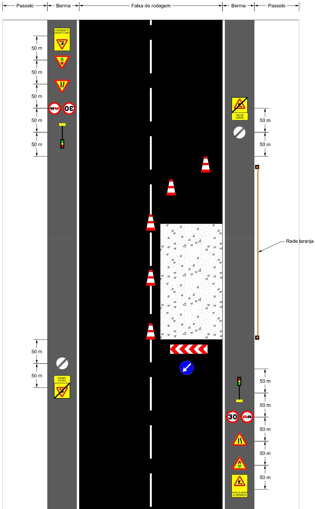
Trabalhos com supressão de uma via - utilização de semáforos de sinalização (dentro de localidade) - com passeio
